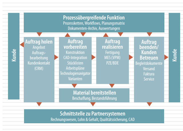
Bild: „Prozesslandkarte“ als Übersicht der in CATUNO.pro enthaltenen Module/Funktionen.
